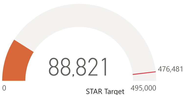
WI-FI Use
