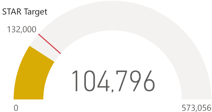
WI-FI Use
